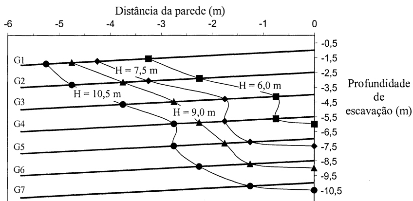
Figura 5 – Localização dos pontos de força axial máxima nos pregos.
