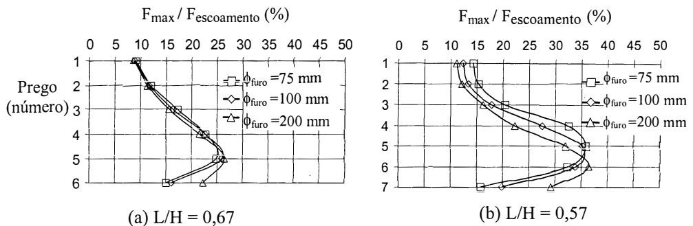
Figura 7 - Influência do diâmetro do furo ( \phi_{\text{furo}} ) nas forças axiais máximas.
