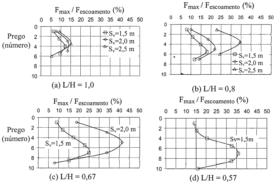
Figura 9 - Influência do espaçamento vertical ( S_v ) nas forças axiais máximas.
