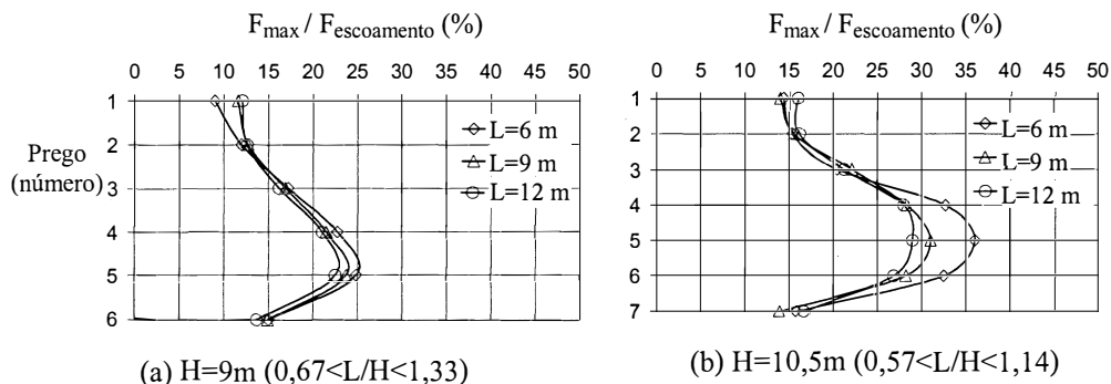
Figura 4 - Influência do comprimento do prego ( L ) nas forças axiais máximas.
