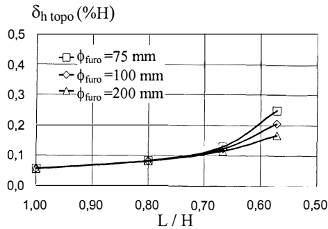
Figura 6 - Influência do diâmetro do furo ( \phi_{\text{furo}} ) nos deslocamentos horizontais ( \delta_{h\text{-topo}} ).
