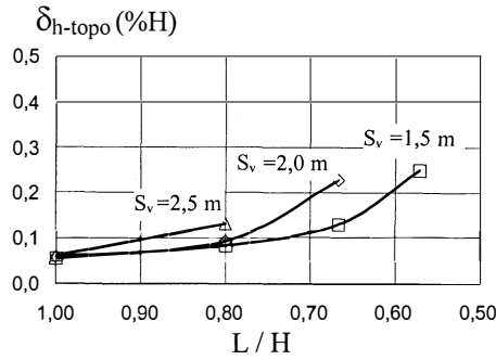
Figura 8 - Influência do espaçamento vertical ( S_v ) nos deslocamentos horizontais ( \delta_{h-topo} ).
