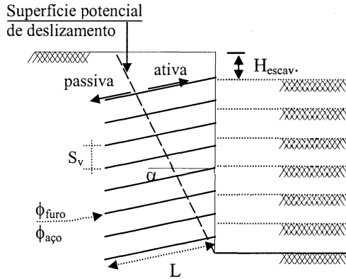
Figura 2 – Mecanismo de ruptura e parâmetros geométricos do muro pregado.
