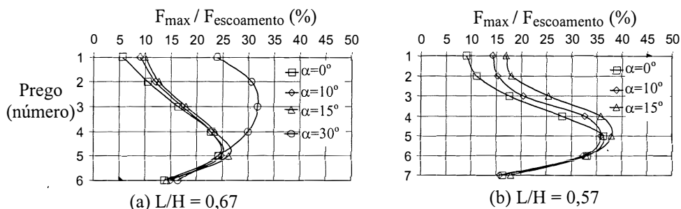
Figura 11 - Influência da inclinação do prego ( \alpha ) nas forças axiais máximas.
