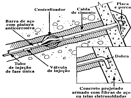
Figura 1 – Esquema de instalação do prego injetado.
