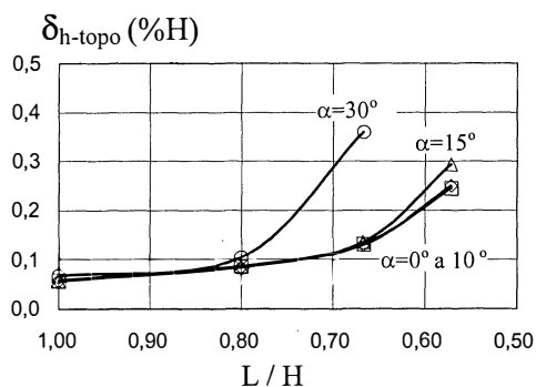
Figura 10 - Influência da inclinação do prego ( \alpha ) nos deslocamentos horizontais ( \delta_{h-topo} ).
