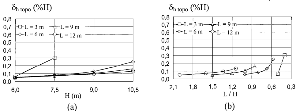
Figura 3 - Influência do comprimento do prego ( L ) nos deslocamentos horizontais ( \delta_{h\text{-topo}} ).
