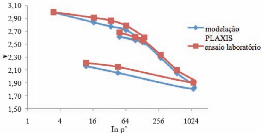
Fig. 3 – Curvas de compressibilidade obtidas no ensaio laboratorial e na modelação realizada no Plaxis, em função de v e \ln p' .
